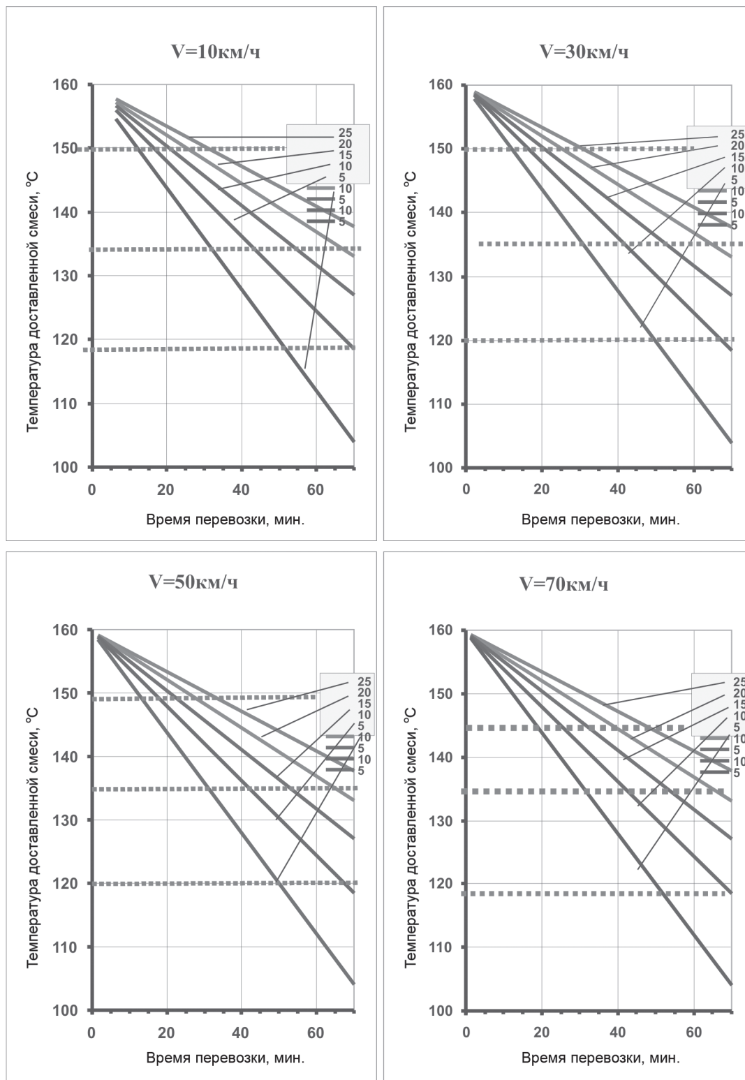
Рисунок В.1 – Время перевозки горячей асфальтобетонной смеси в автомобилях самосвалах (при температуре отгрузки t_{нач} = 160 \text{ } ^\circ\text{C} )
