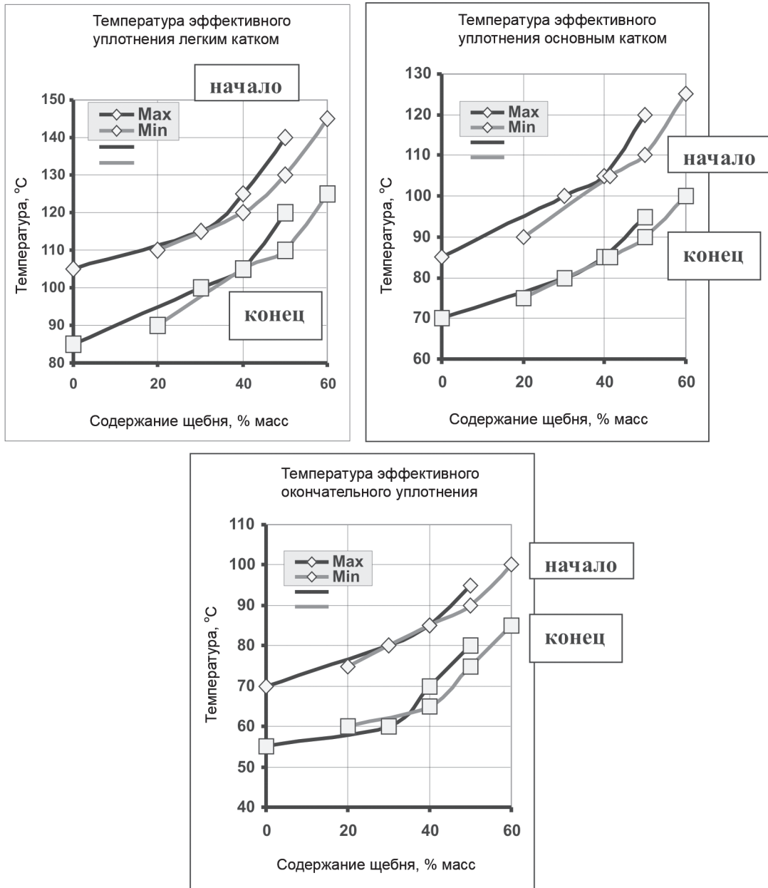
Рисунок Г.1 – Определение температуры эффективного уплотнения асфальтобетонных смесей на различных этапах работы звена дорожных катков
